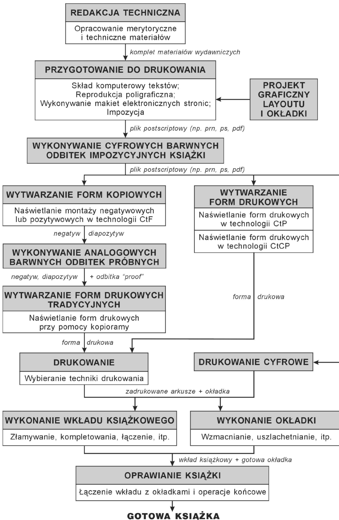
Rys. 2. Przykładowy schemat blokowy obrazujący procesy technologiczne wytwarzania książki – z możliwością zastosowania alternatywnych „ścieżek” produkcji
